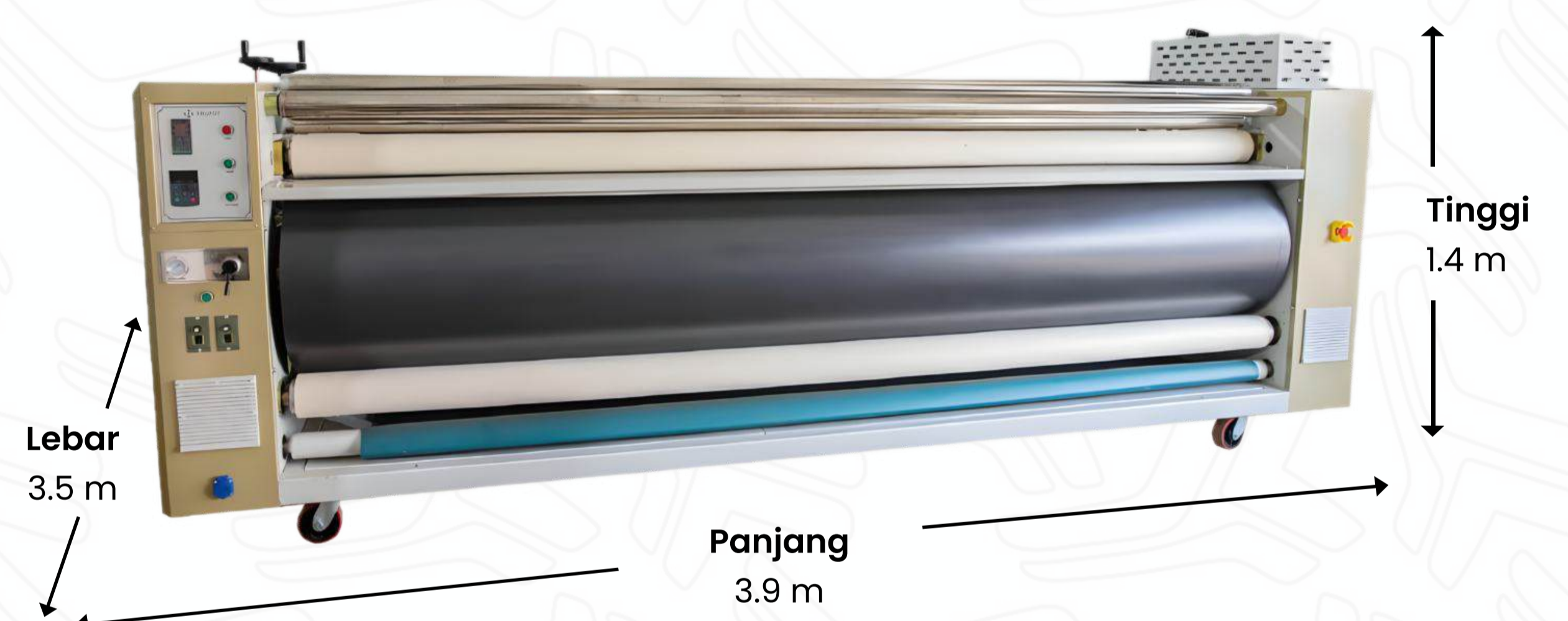
Ukuran Mesin Roll Heat Press ZH3242
